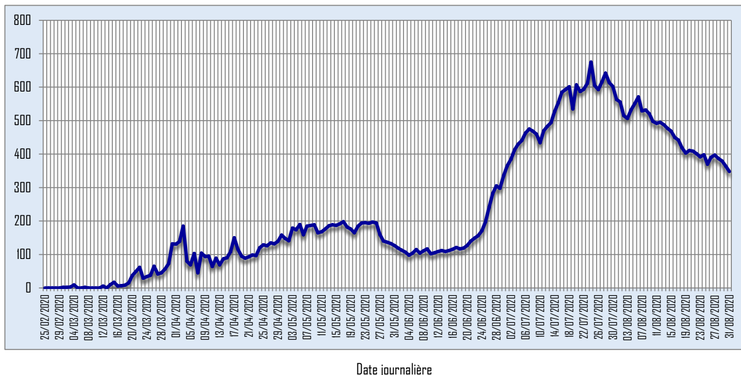
Fig 5 : Situation épidémiologique de l'infection au nouveau coronavirus SARS Cov 2 Evolution des cas incidents journaliers en histogramme – Algérie au 31 Août 2020
