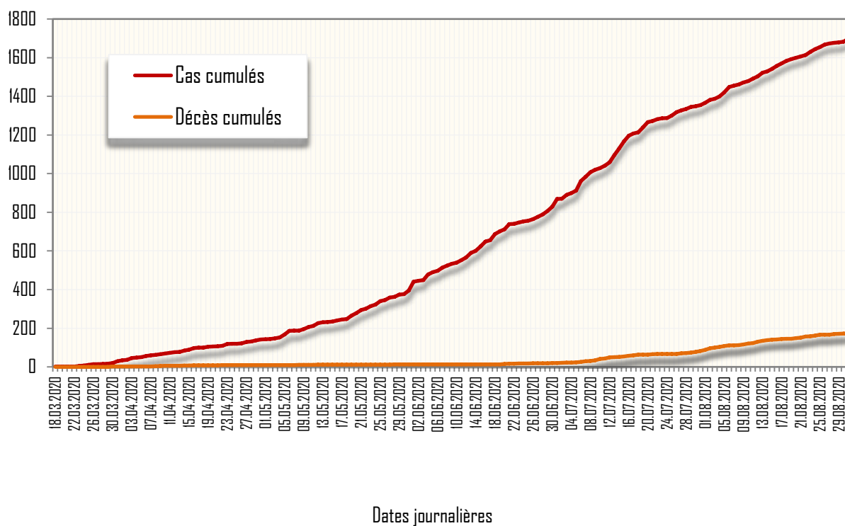
Fig 33 : Situation épidémiologique de l'infection au nouveau coronavirus Evolution des courbes de la distribution des fréquences d'infections à coronavirus cumulés et des décès cumulés – EHUO au 31 Août 2020
