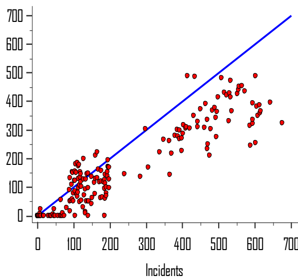
Fig 11 : Situation épidémiologique de l'infection au nouveau coronavirus SARS Cov 2 – Diagramme d'un nuage de point mettant la relation de l'évolution des cas incidents journaliers en fonction des cas rétablis - Algérie au 31 Août 2020
