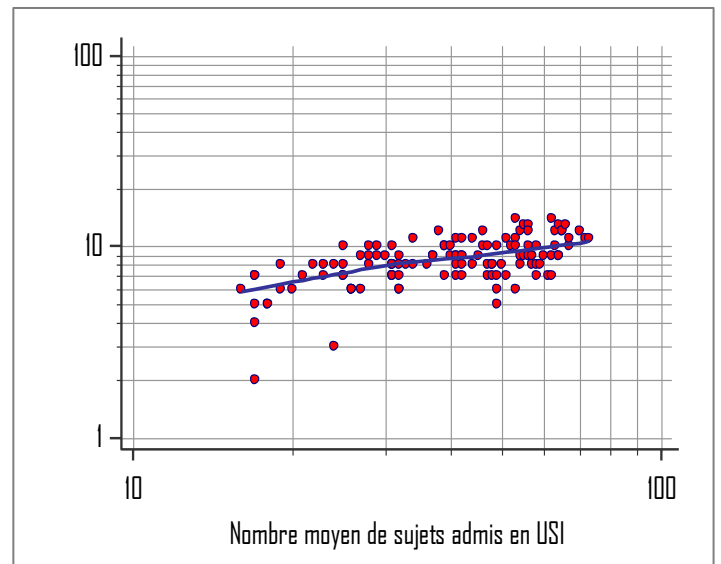
Fig 18 : Situation épidémiologique de l'infection au nouveau coronavirus SARS Cov 2 – Diagramme avec nuage de points de la Correlation entre le nombre de décès et le nombre moyens de cas admis en USI - (Echelle logarithmique) Algérie au 31 Août 2020
