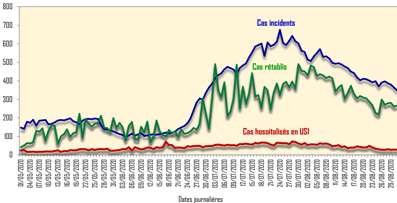
Fig 10 : Situation épidémiologique de l'infection au nouveau coronavirus SARS Cov 2 – Evolution des cas incidents journaliers, cas guéris et sujets admis en USI - Algérie au 31 Août 2020
