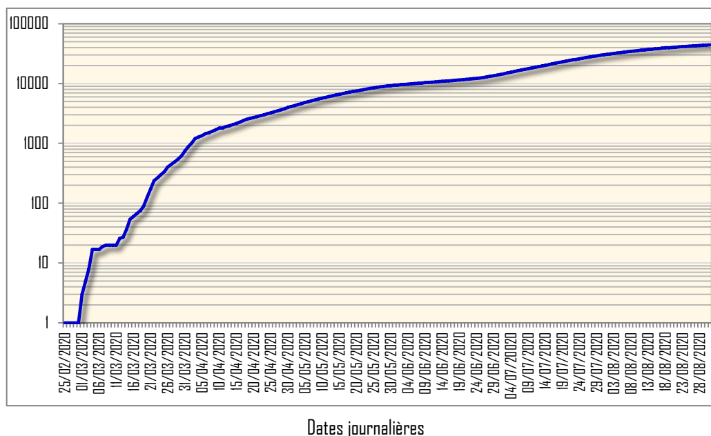
Fig 9 : Situation épidémiologique de l'infection au nouveau coronavirus SARS Cov 2 Evolution logarithmique des cas incidents journaliers cumulé en polygone de fréquence absolue – Algérie au 31 Août 2020
